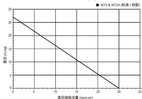
真空度-真空抽吸流量对比 入口压力为70-110psig
