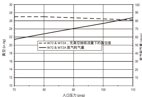
真空度及氮气耗气量-入口压力对比
